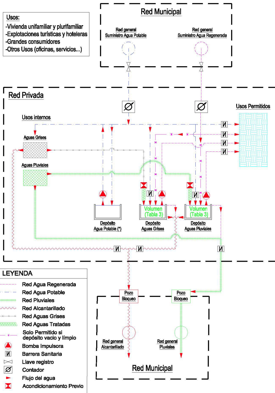
FIGURA 1. ESQUEMA INSTALACIÓN AGUAS GRISES, REGENERADAS Y PLUVIALES
